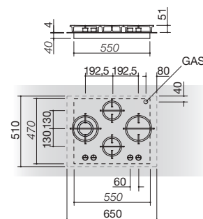
Mood da 65 per profondità 51 3 gas + 1 doppia corona Flat Eco-Design (lunghezza piano 65)
