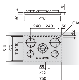
Mood da 75 per profondità 51 4 gas + 1 doppia corona Flat Eco-Design (lunghezza piano 75)
