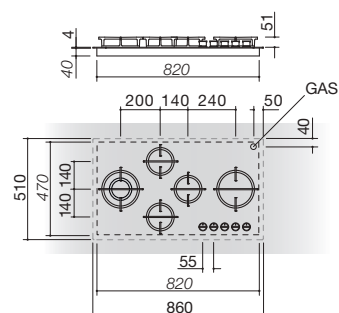
Mood da 90 per profondità 51 4 gas + 1 doppia corona Flat Eco-Design (lunghezza piano 95)
